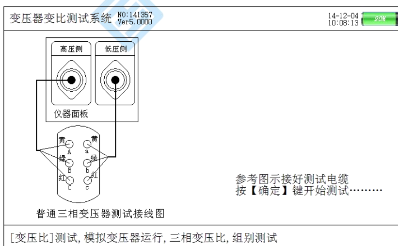
图 6 三相变压比测试接线提示屏
