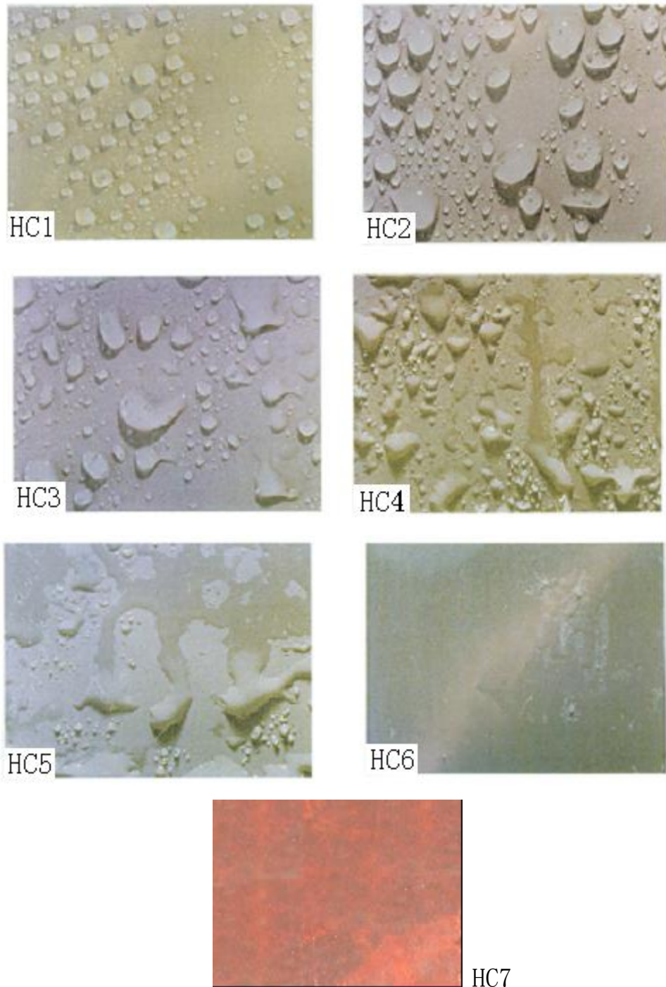
图 3 不同憎水等级的 STRI 标准图象
